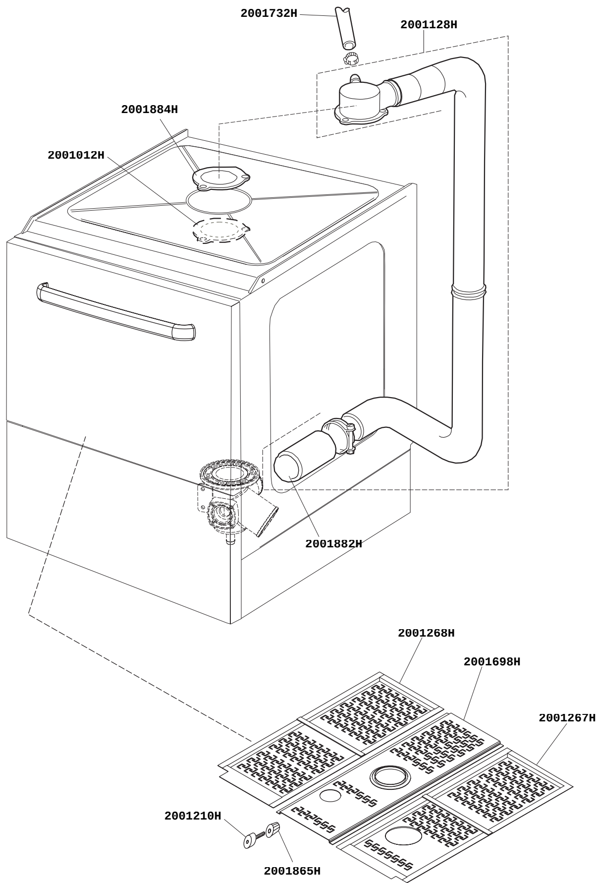
Filtres Inox
